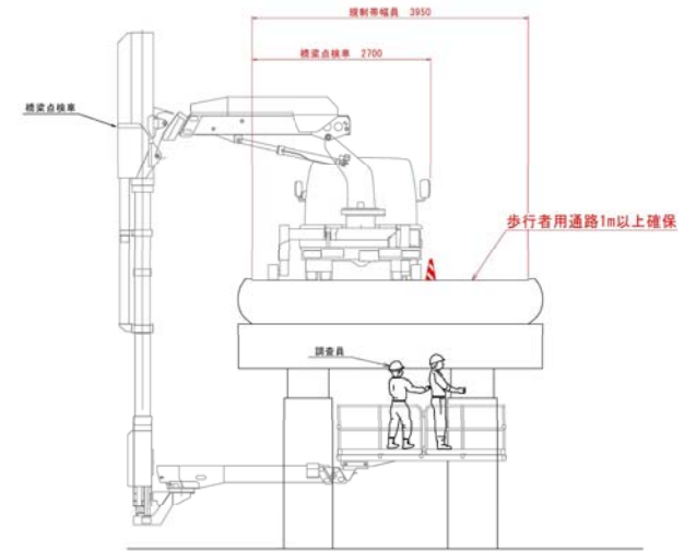
規制帯断面図 (時間止め通行規制)
